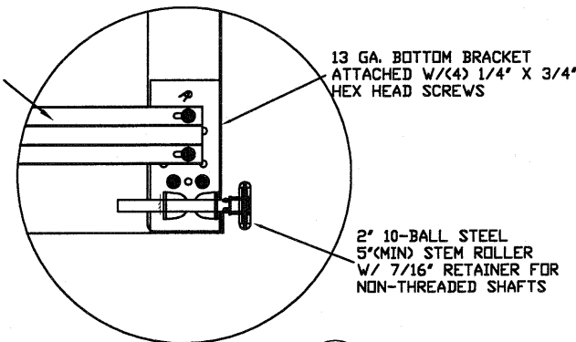
TYPICAL BOTTOM BRACKET N.T.S. ⑤
